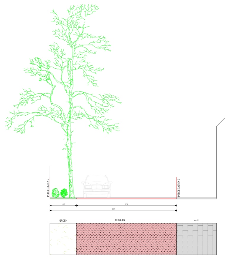
Dwarsprofiel 4 Bergstraat
