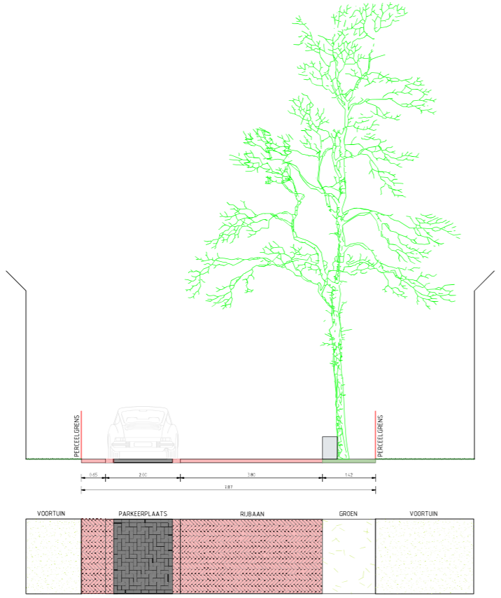
Dwarsprofiel 6 Bergstraat
