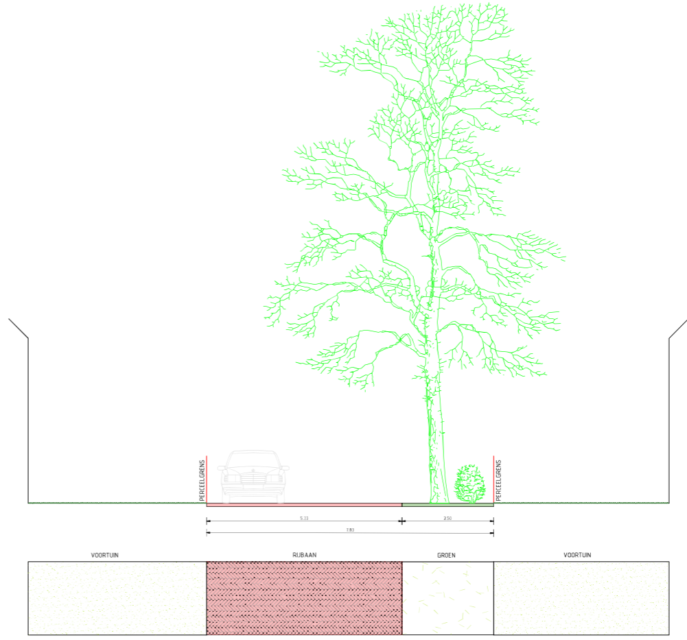
Dwarsprofiel 5 Bergstraat
