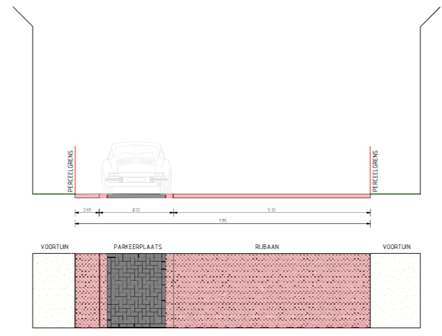
Doorsnede 3 Ennstraat
