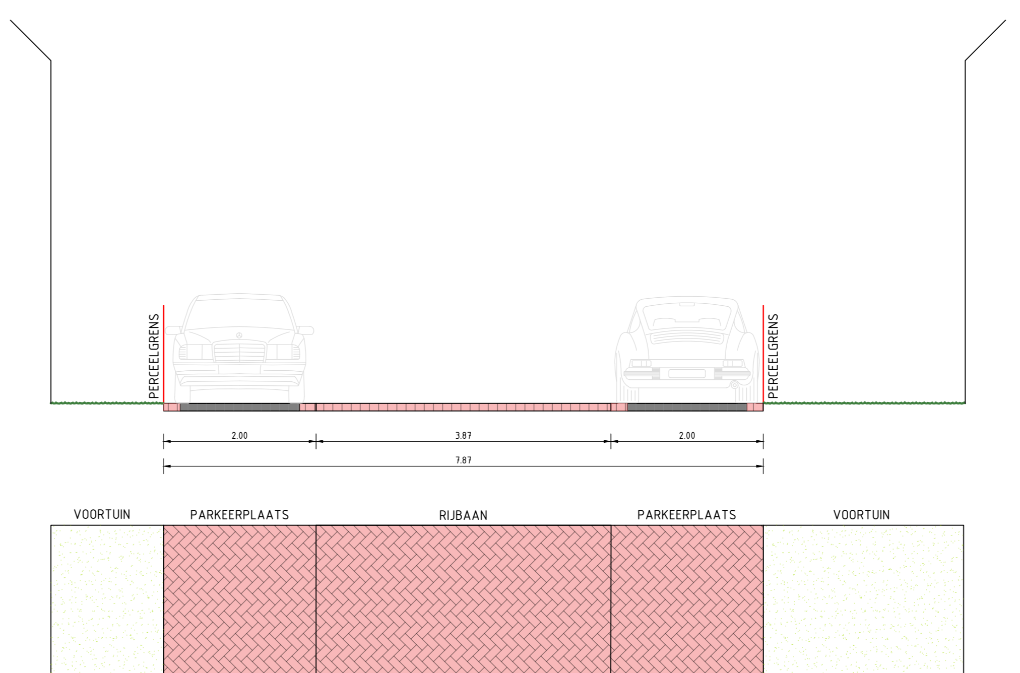
Dwarsprofiel 6 Bergstraat
