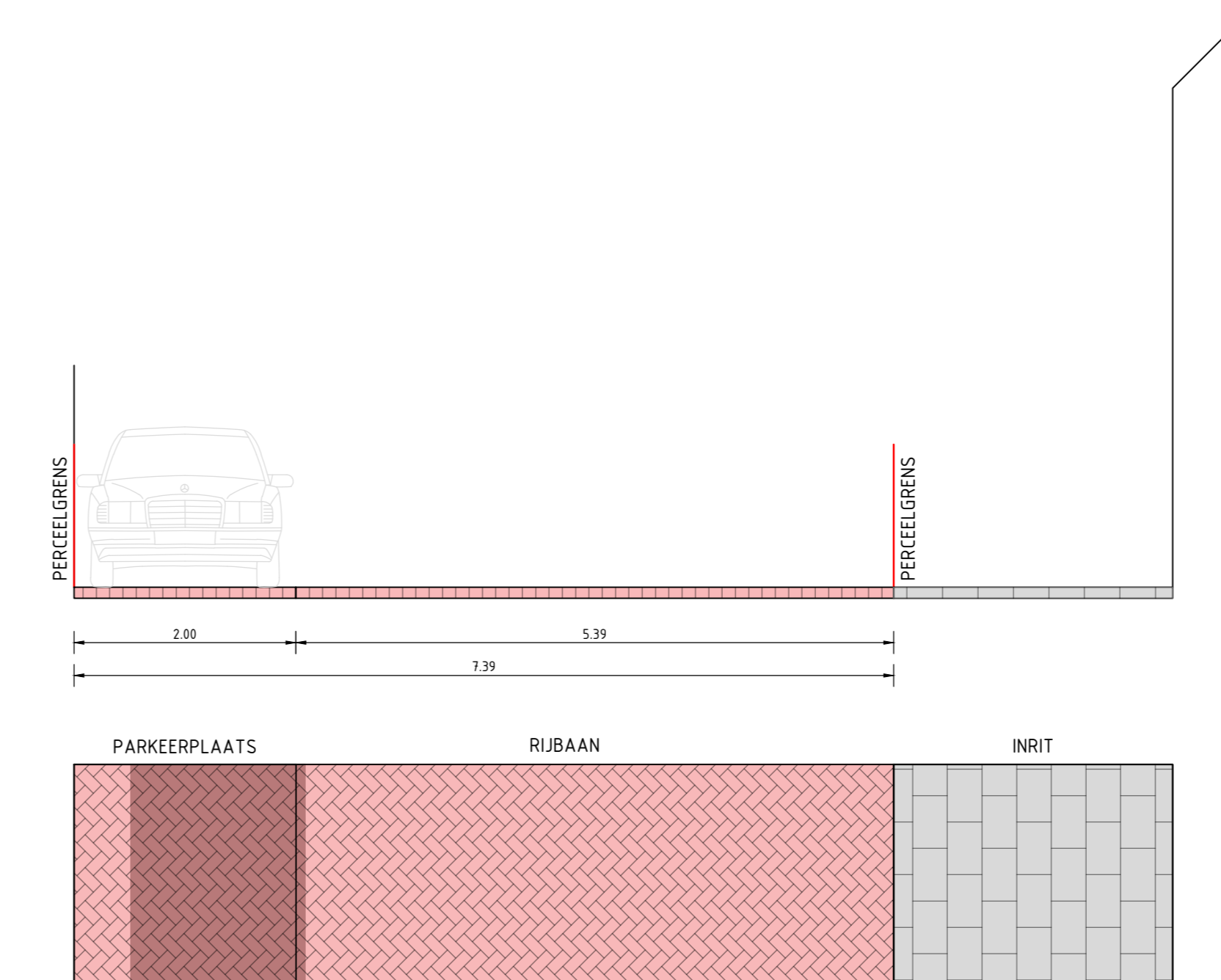
Dwarsprofiel 4 Bergstraat
