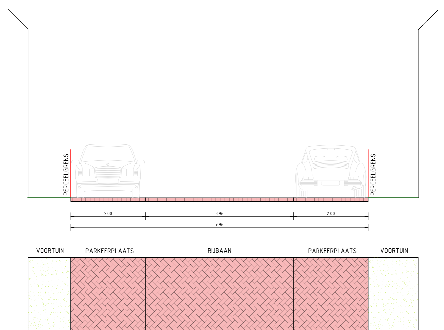
Dwarsprofiel 1 Emmastraat
