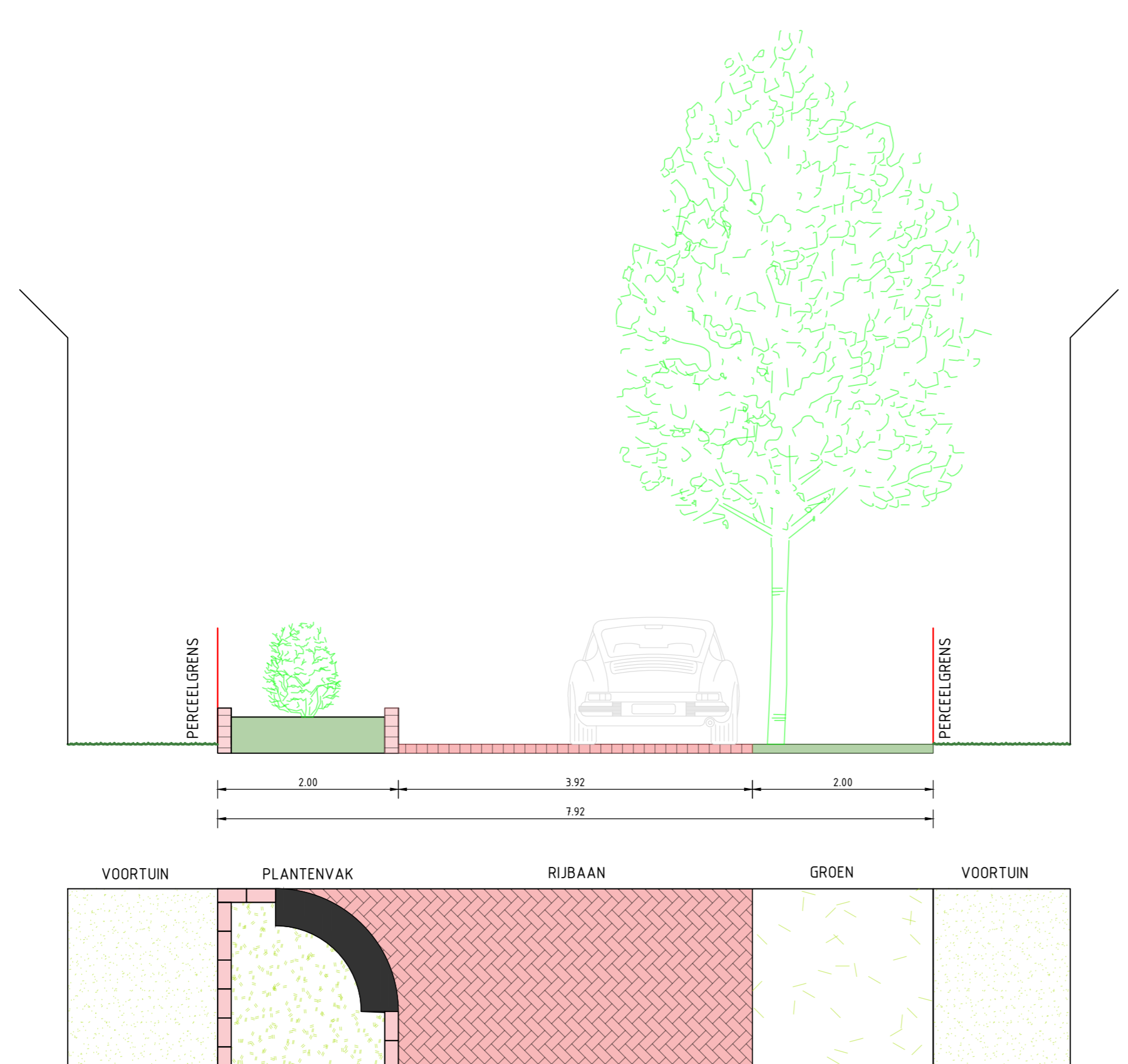
Dwarsprofiel 3 Emmastraat
