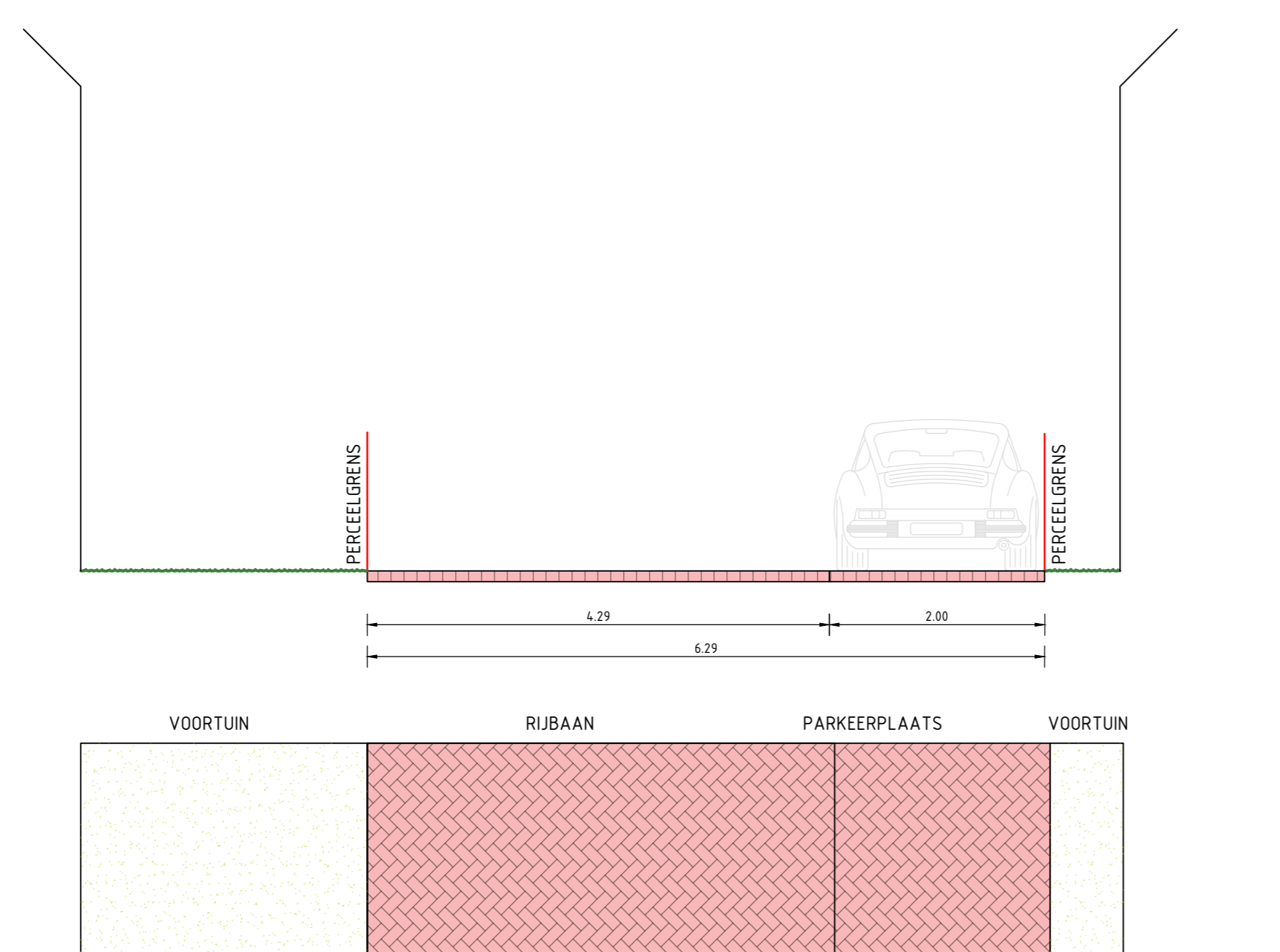
Dwarsprofiel 2 Emmastraat
